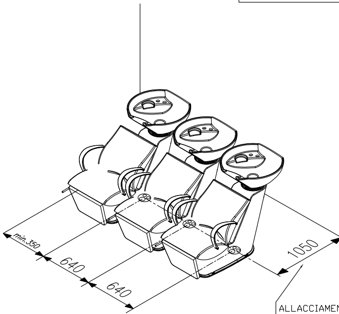
ALLACCIAMENTO IDRAULICO HYDRAULIC CONNECTION
