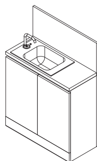
4 50832 MODULO LAVABO 80 WASHBASIN MODULE ↑ 1130 mm ↗ 400 mm → 800 mm
